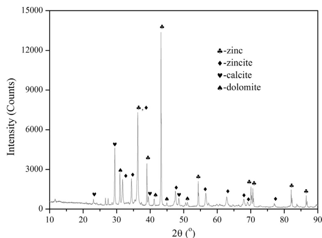
Fig. 1. XRD pattern of the ZPR.
