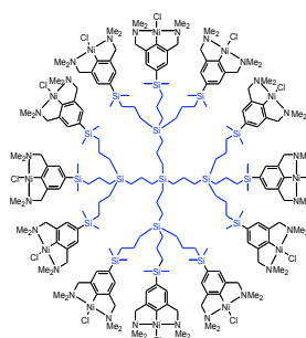
1994, CS-(NCN-NiX)_{12}
