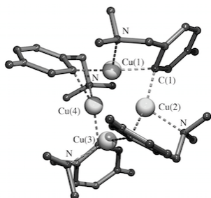
1972, R_4Cu_4
